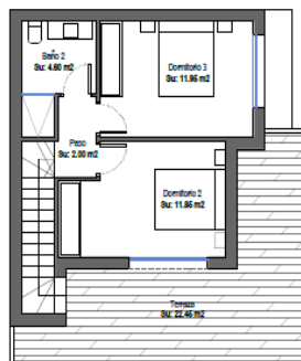
Planta Primera
